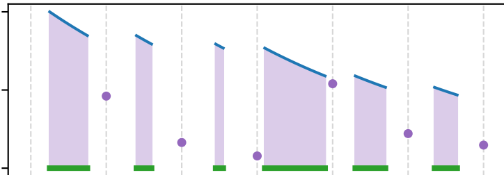
Raw data
